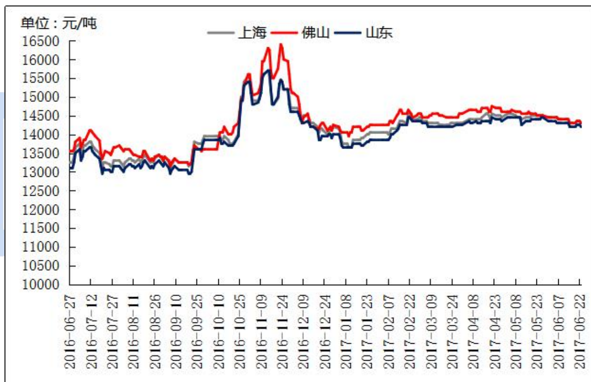
图六、全国主流地区A356.2铝合金锭价格走势 规格：国标
