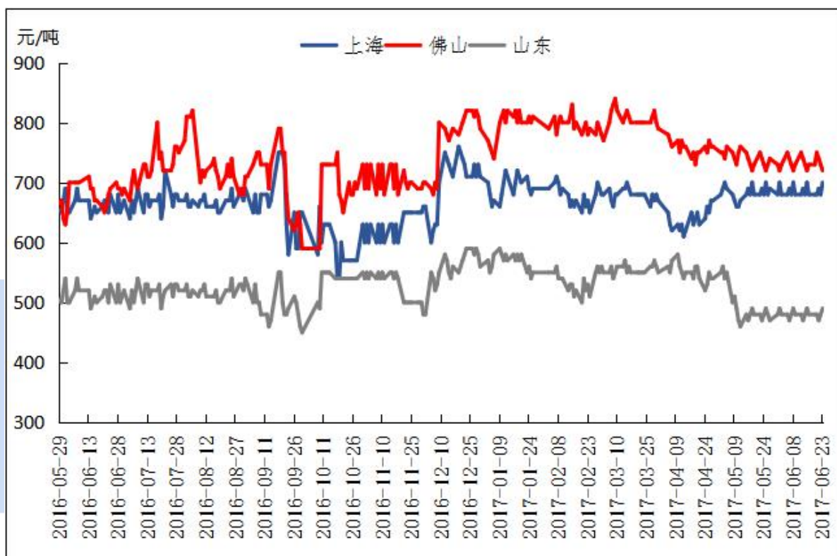
图七、全国主流地区 A356.2 铝合金锭加工费走势图 规格：国标
