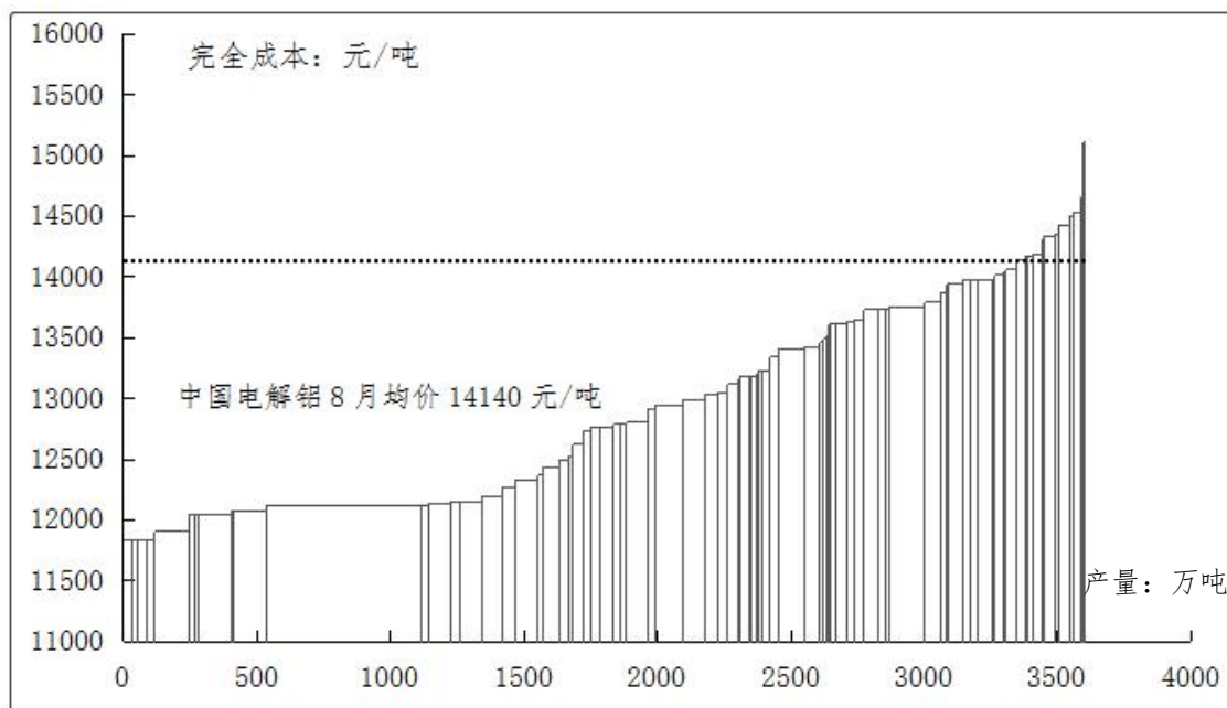
图 10、国内电解铝行业成本曲线（完全成本）
