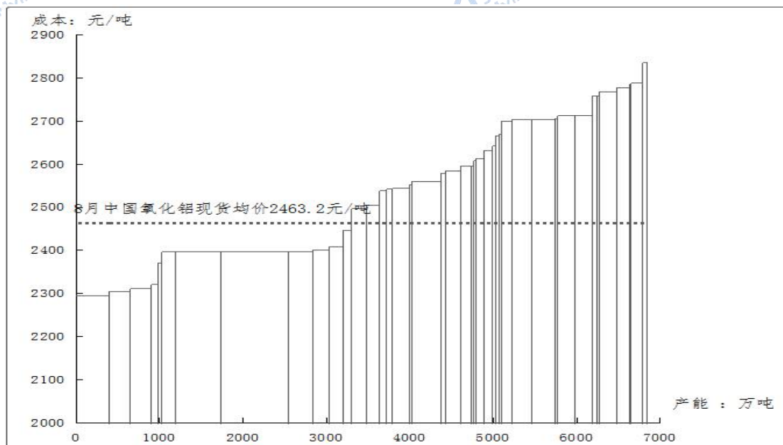
图 5、国内氧化铝行业成本曲线（完全成本）
